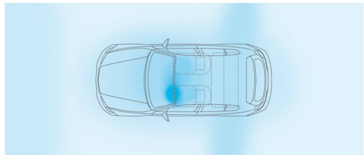
VEGA-11 / mesures du champ de torsion (aiguille)
