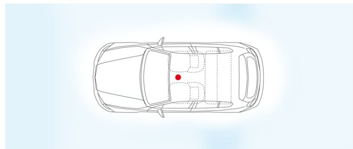
Champ de torsion gauche
